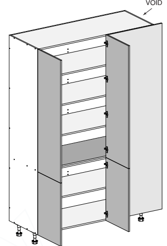
2 DOOR - SPLIT
