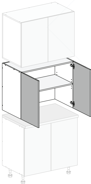
2 DOOR
