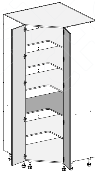
2 DOOR - ANGLE
