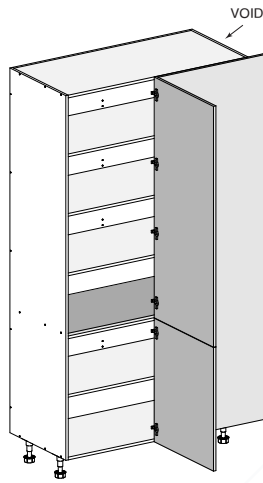
1 DOOR - SPLIT
