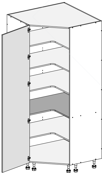
1 DOOR - ANGLE
